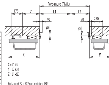
Porta con CP2 o RC2 non apribile a 180°
