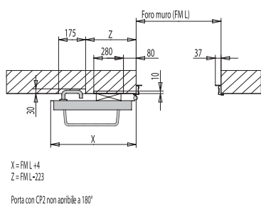
Porta con CP2 non apribile a 180°
