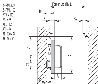
Ingombri massimi per porte ad una anta con apertura a 90°.
