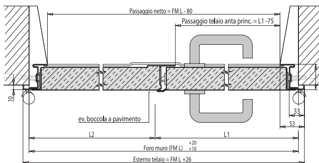
Sezione orizzontale Unirev REI 60 / REI 120 a due ante
