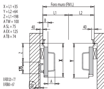
Ingombri massimi per porte a due ante con apertura a 90°.
