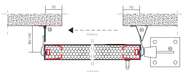
Particolare inferiore ROTEO SILVER montato oltre luce ad una anta, asse 90 / 140 mm
