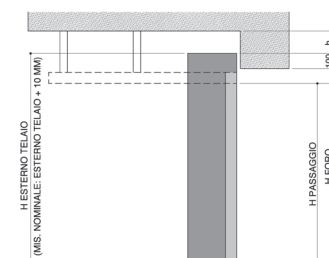
POSIZIONE OLTRE LUCE STRUTTURA SIKURA CITY HF
