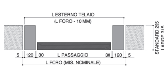
POSIZIONE IN LUCE STRUTTURA SIKURA CITY HF
