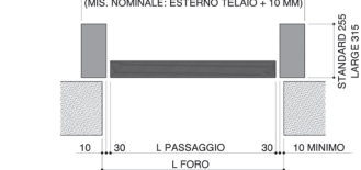
POSIZIONE OLTRE LUCE STRUTTURA SIKURA CITY HF
