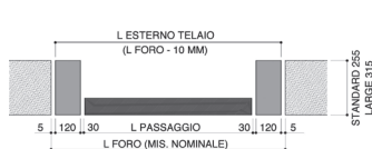
POSIZIONE IN LUCE STRUTTURA SIKURA CITY HF
