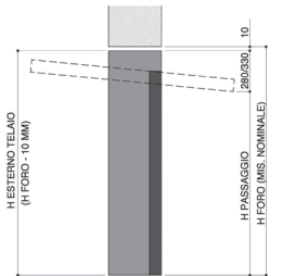
POSIZIONE IN LUCE STRUTTURA SIKURTEC HF
