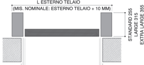
POSIZIONE OLTRE LUCE STRUTTURA SIKURA HF
