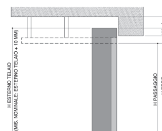
POSIZIONE OLTRE LUCE STRUTTURA SIKURA CITY HF
