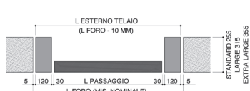
POSIZIONE IN LUCE STRUTTURA SIKURA HF
