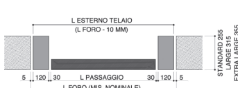
POSIZIONE IN LUCE STRUTTURA SIKURA CITY HF
