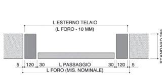
POSIZIONE IN LUCE STRUTTURA SIKURTEC CITY HF
