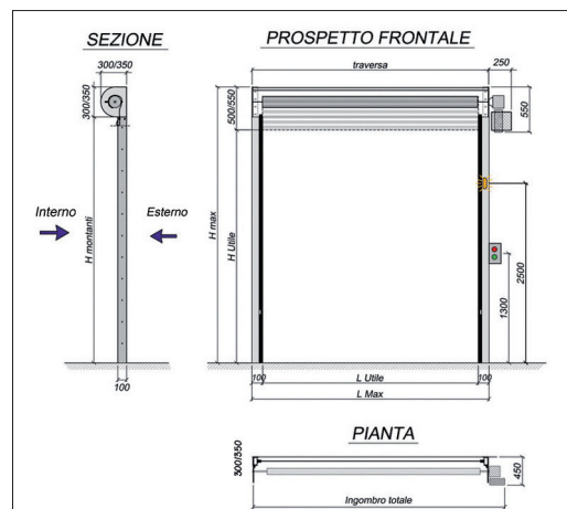
Disegni tecnici portone rapido Eolo Interior.
