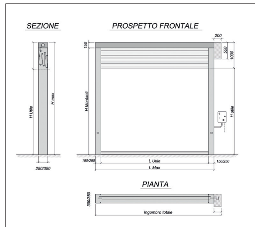
Disegni tecnici portone rapido Eolo Impac.
