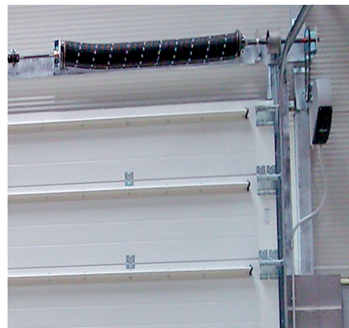
Porta sezionale industriale con motorizzazione. In evidenza i rinforzi orizzontali che vengono sempre inseriti nelle porte di grandi dimensioni.
