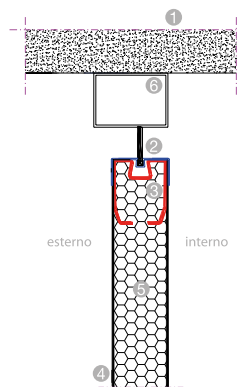
Particolare superiore portone ALISEO montato in luce
