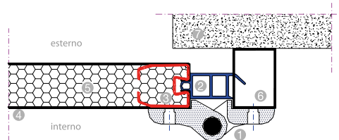
Particolare laterale ALISEO applicato oltre luce
