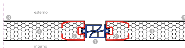
Particolare incontro centrale ALISEO
