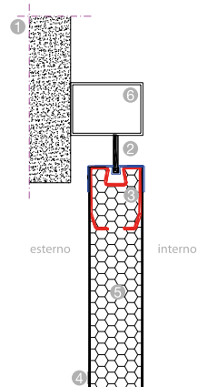
Particolare superiore portone ALISEO montato oltre luce
