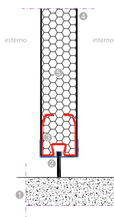
Particolare inferiore portone ALISEO
