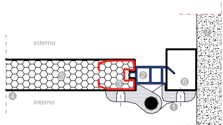
Particolare laterale ALISEO applicato in luce
